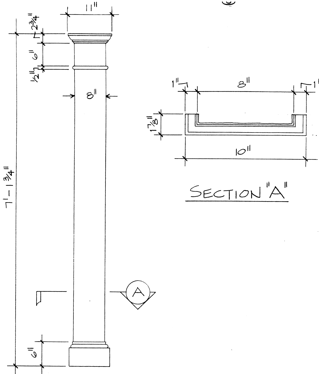
ELEVATION
